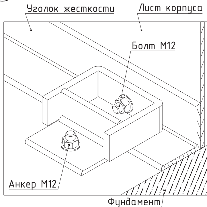
13 Комплект креплений к фундаменту
